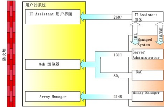
图 11-1. 防火墙后面的典型安装
